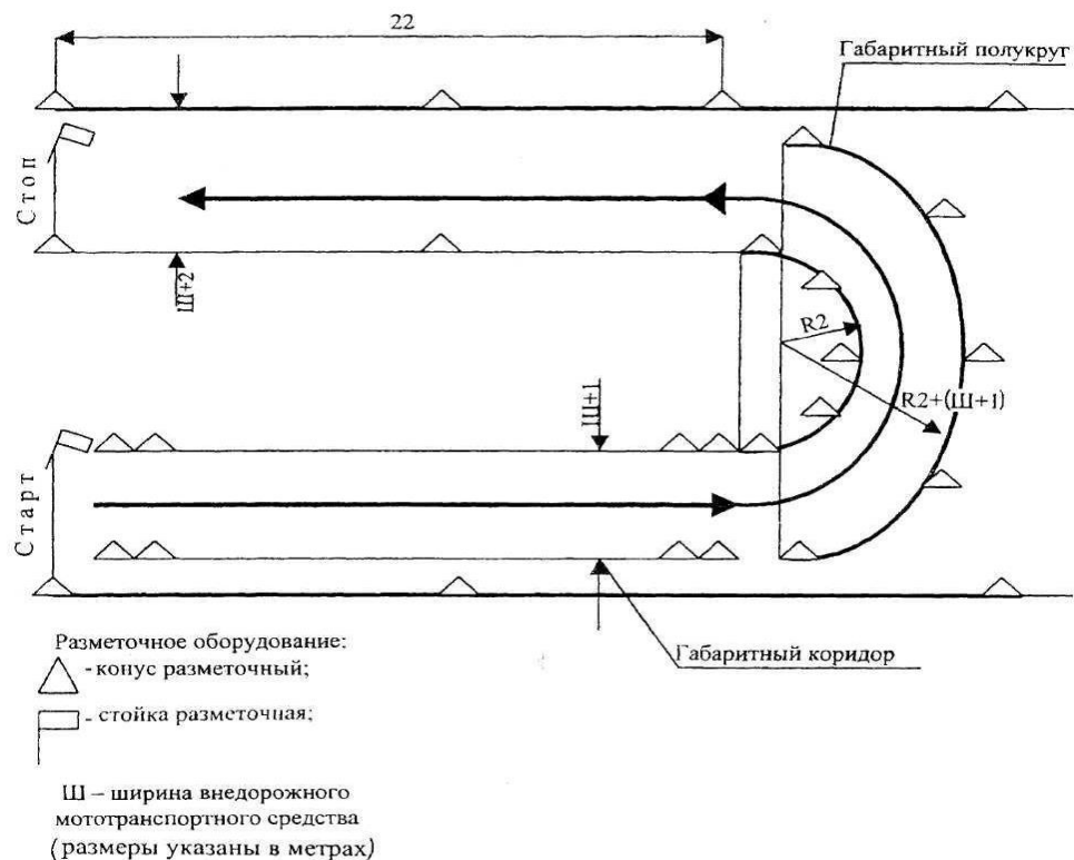
Рис. 2. Габаритный коридор, габаритный полукруг, разгон-торможение
